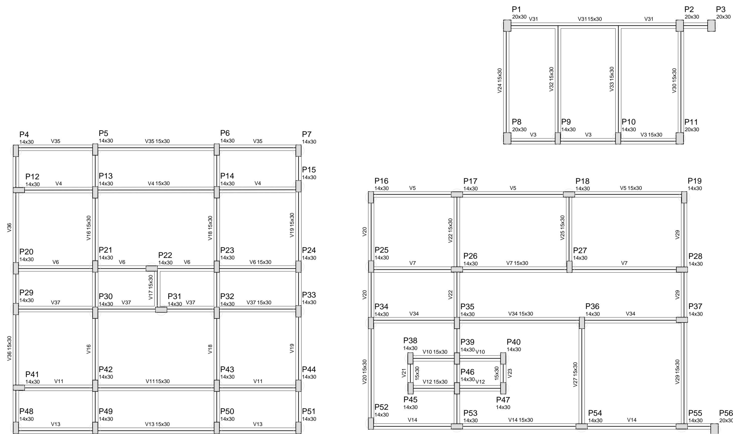
Forma do pavimento BALDRAME ESCALA 1:50
