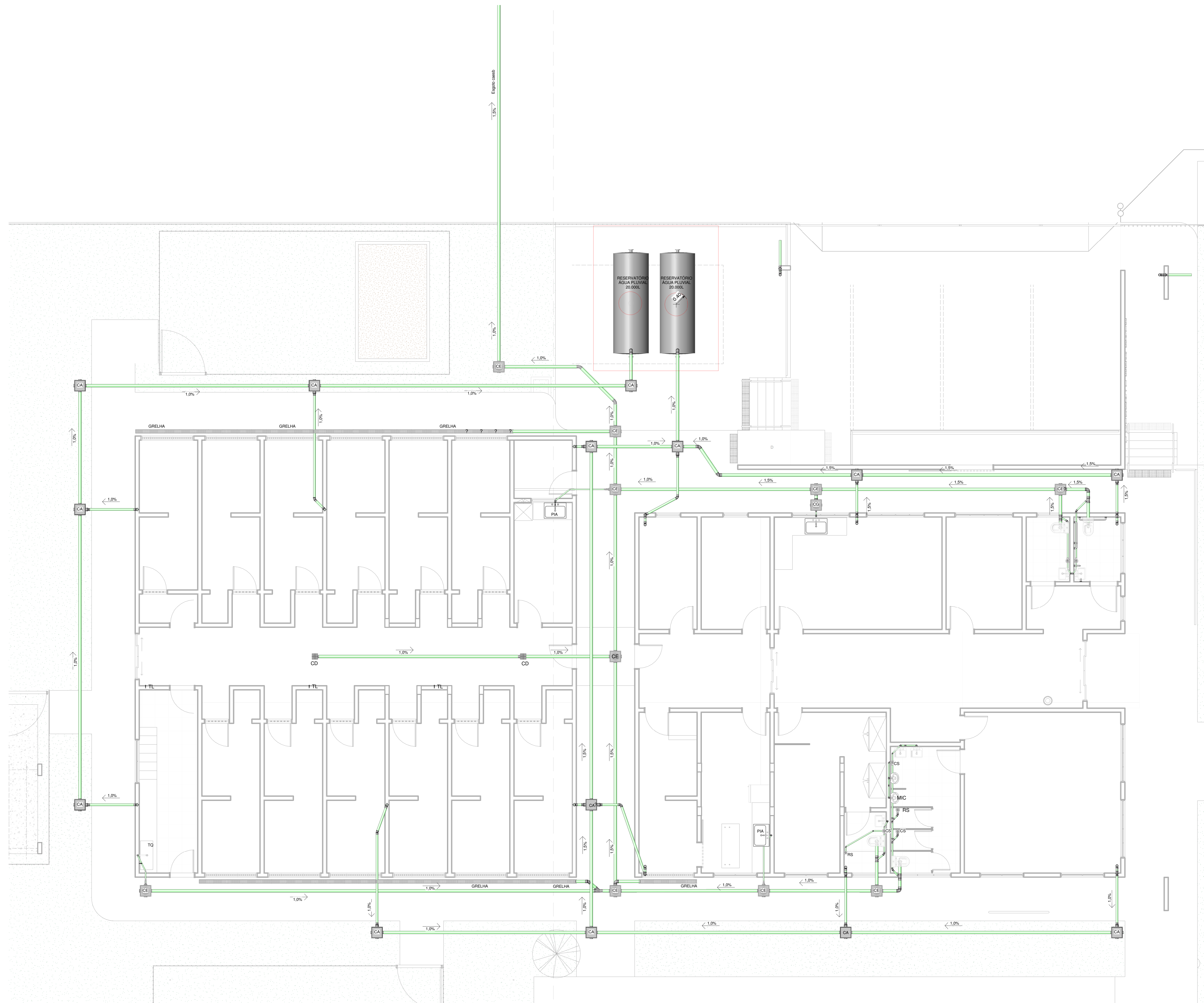
1 ESGOTO 1:50
