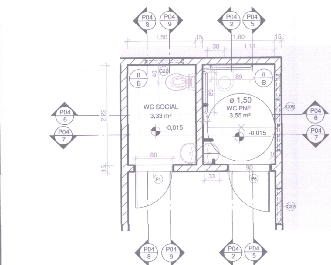
1 DET. WC PNE ESCALA 1:50
