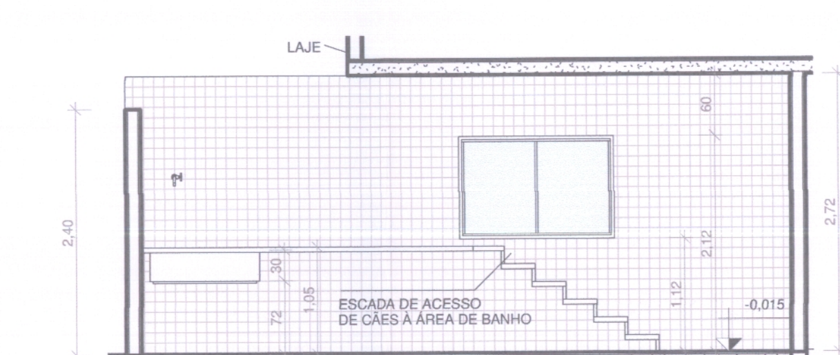
19 DET. BANHO CANIL - AA1 ESCALA 1:50
