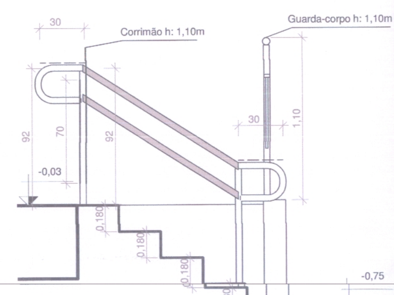
4 DET. ESCADA ESCALA 1:25
