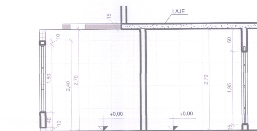
23 DET. BOX CANIL - AA1 ESCALA 1:50
