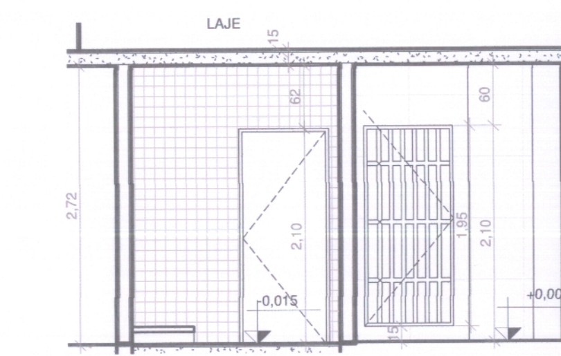
21 DET. BANHO E BOX - BB1 ESCALA 1:50
