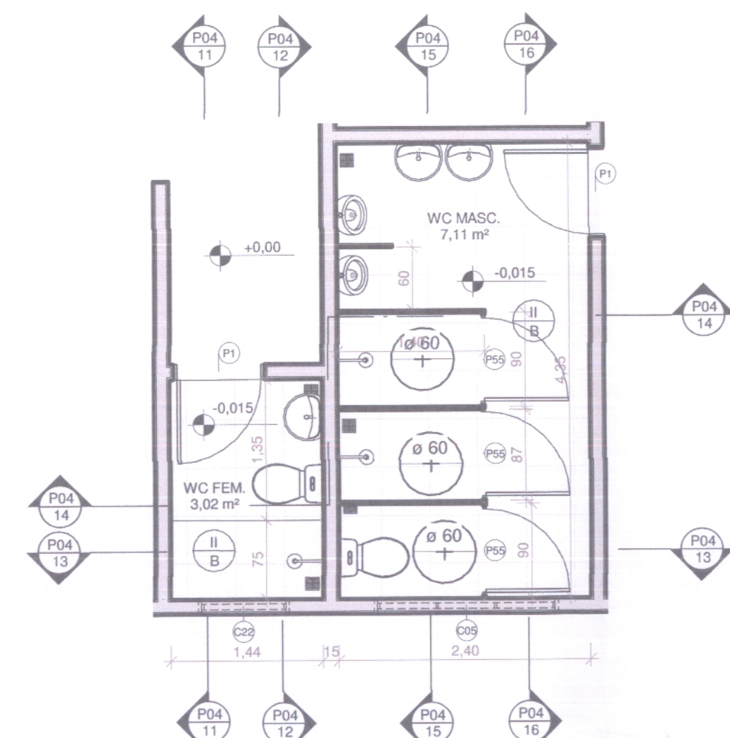
10 DET. WC MASC. E FEM. ESCALA 1:50
