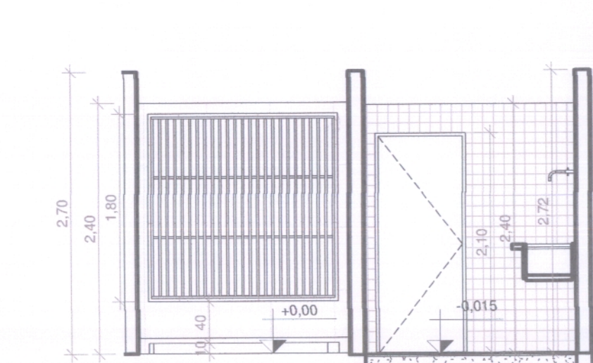
22 DET. BANHO E BOX - BB2 ESCALA 1:50
