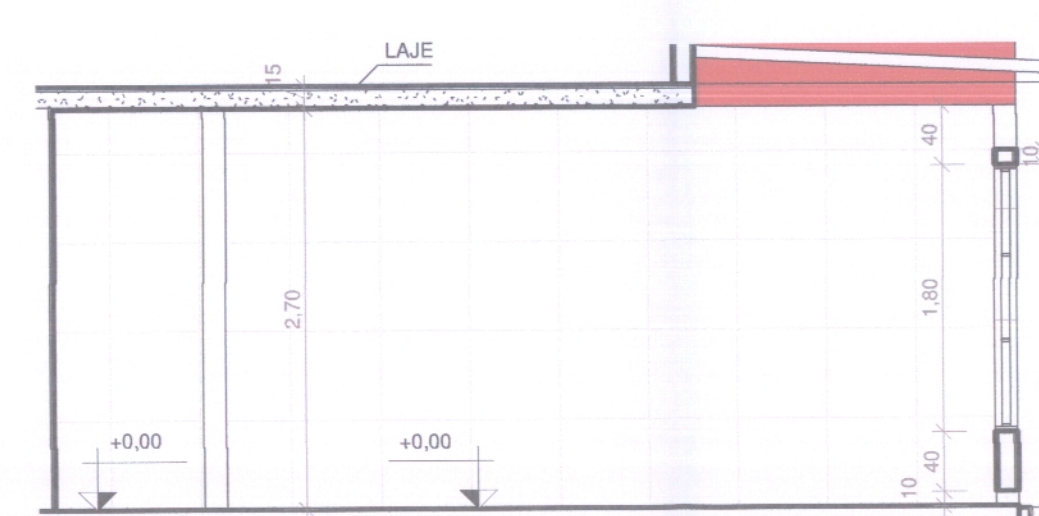
24 DET. BOX CANIL - AA2 ESCALA 1:50
