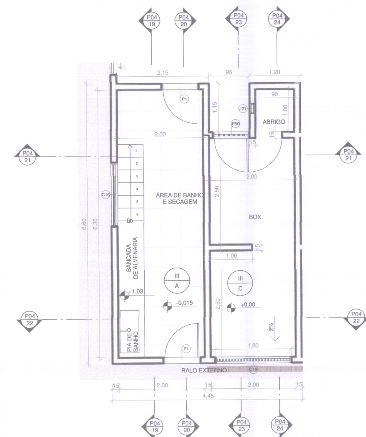
19 DET. BANHO CANIL - AA1 ESCALA 1:50
