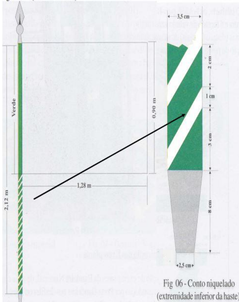
Figura 06 – (modelo de haste)
