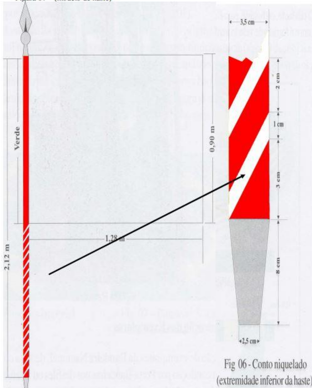
Figura 07 – (modelo de haste)
