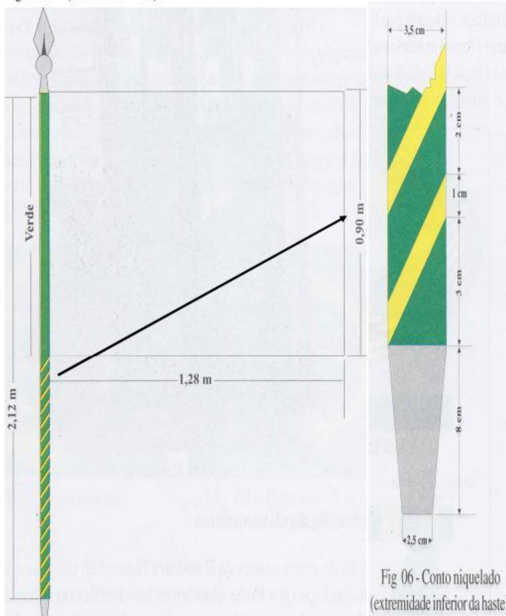
Figura 05 – (modelo de haste)
