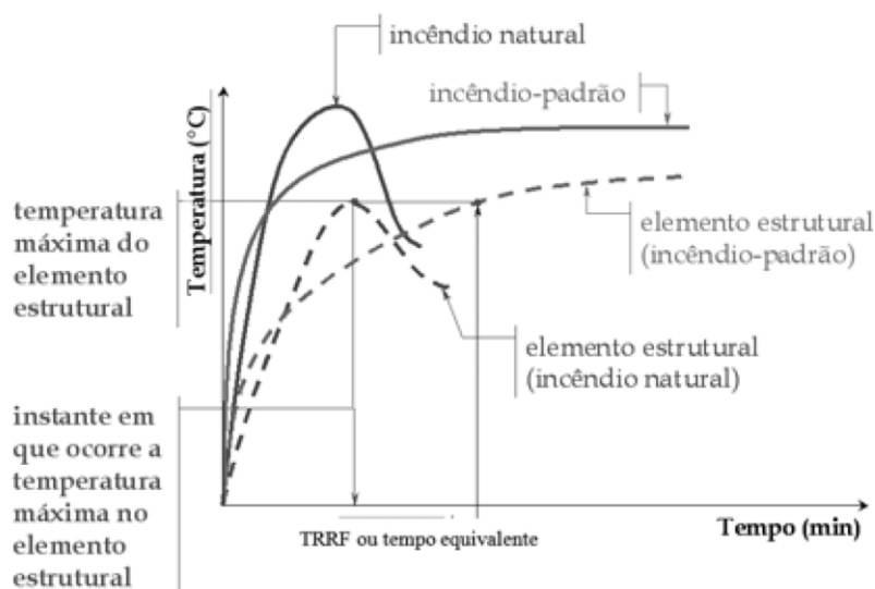
Figura 71 - Comparativo entre as curvas modelo e as curvas reais
