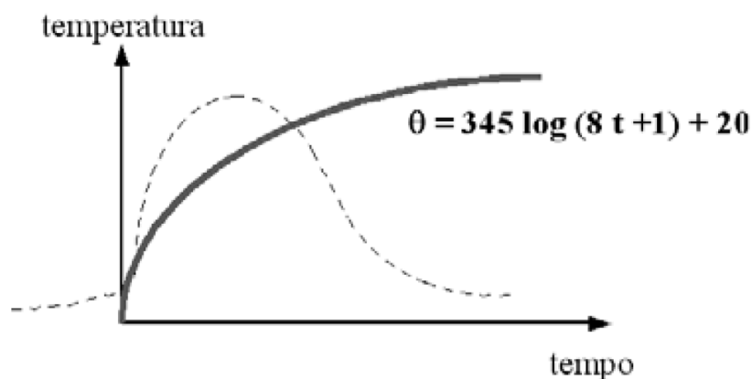
Figura 66 - Curva modelo para o Incêndio Padrão
