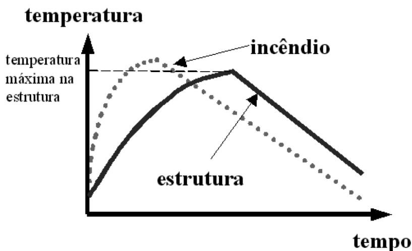
Figura 68 - Temperatura máxima na estrutura
