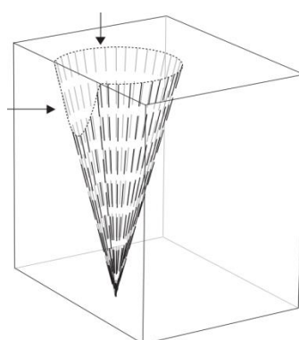
Figura 36 - Padrão de queima em U
