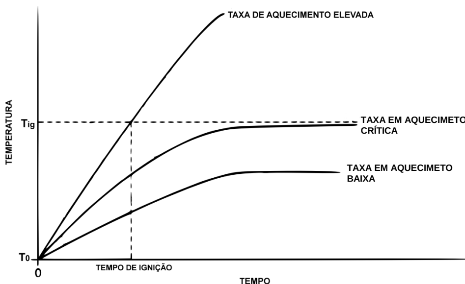
Figura 14 - Curva de crescimento em temperatura de um material com o tempo.
