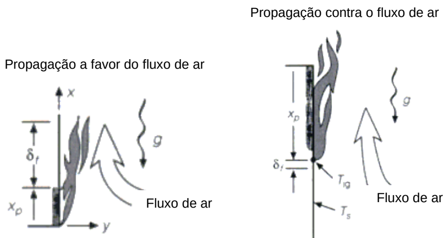
Figura 20 - Propagação vertical da chama a favor e contra o fluxo de ar
