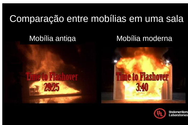
Figura 28 - Comparação do comportamento do incêndio com mobiliário antigo e com moderno
