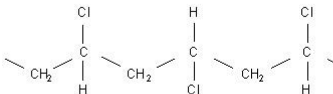
Figura 3 - Estrutura do pvc
