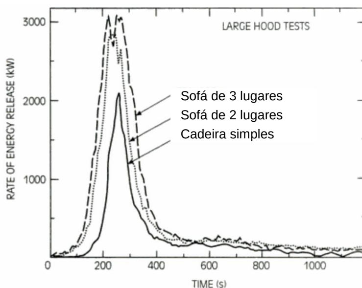
Figura 23 - Curva da Taxa de liberação de calor pelo tempo para diversos tipos de mobiliário.
