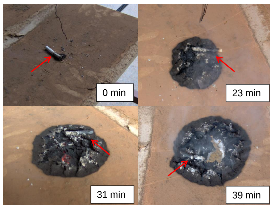
Figura 17 - Fotos da propagação do fogo devido ao cigarro sobre a placa de papel prensado. A seta identifica o cigarro
