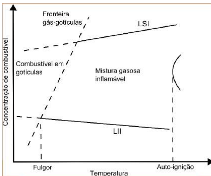
Figura 12 - relação entre limite de inflamabilidade, temperatura e concentração do combustível
