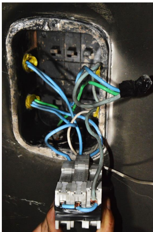
Figura 86 - Sistemas de proteção elétrica da edificação
