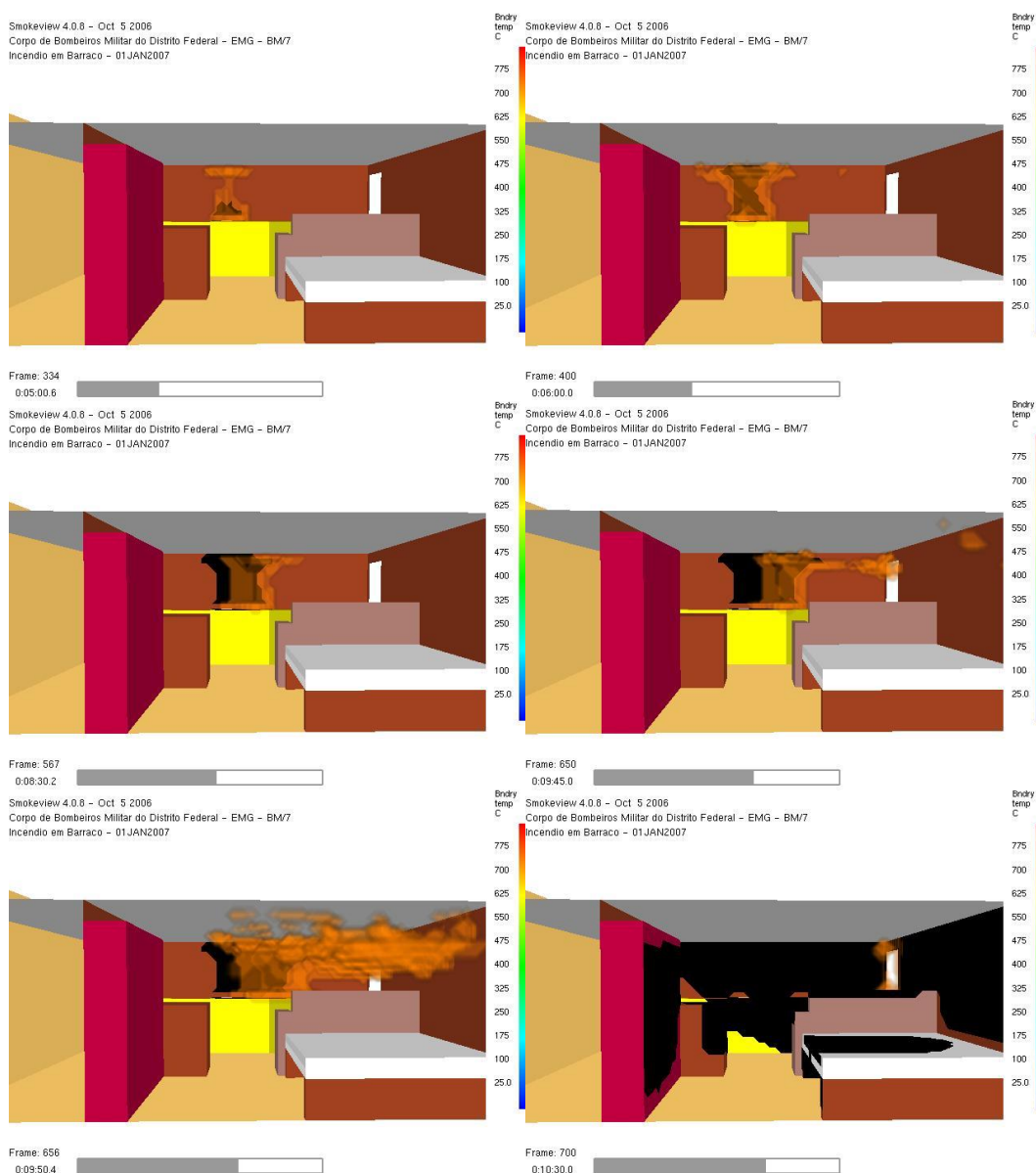
Figura 47 - Influência da criação nas marcas de queima devido à ventilação natural (porta aberta). Simulação computacional realizada em um incêndio real periciado pelo CBMDF
