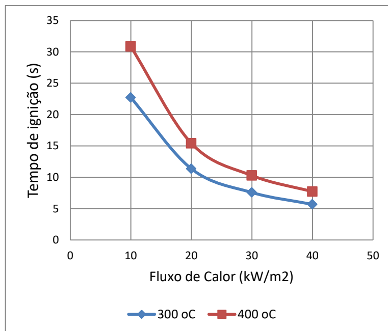
Figura 19 - Gráfico do tempo de ignição (Exercício 3)
