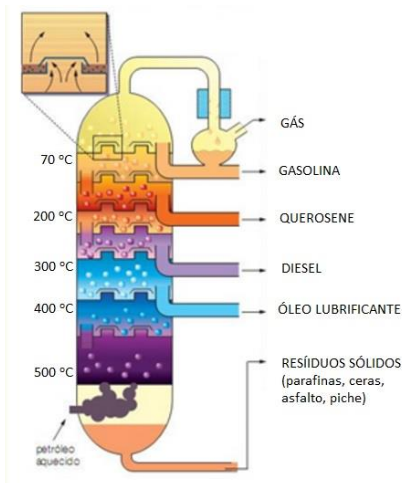
Figura 13 - Frações do petróleo
