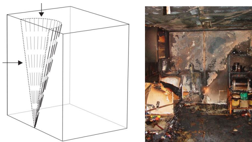
Figura 35 - Padrão de queima em V ou cone
