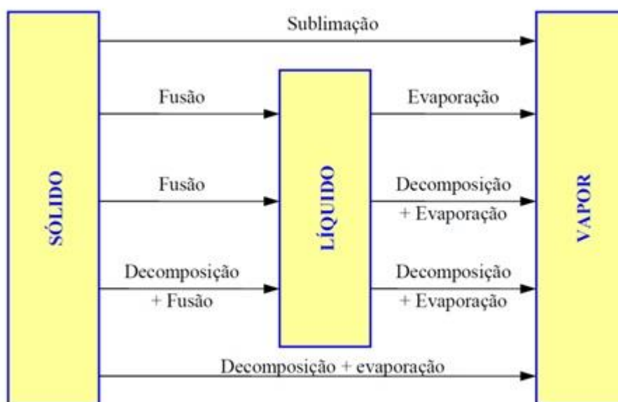
Figura 5 - Diferentes maneiras que o vapor inflamável pode ser gerado de um combustível sólido
