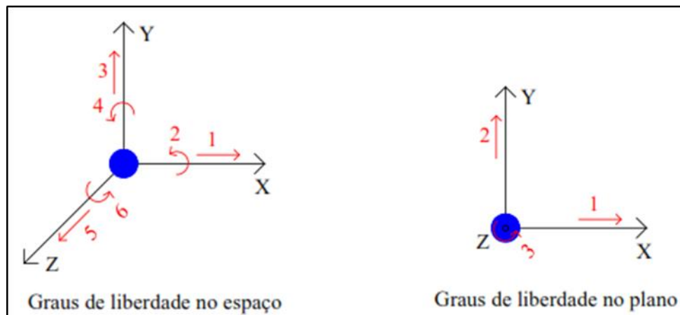
Figura 55 - Graus de liberdade
