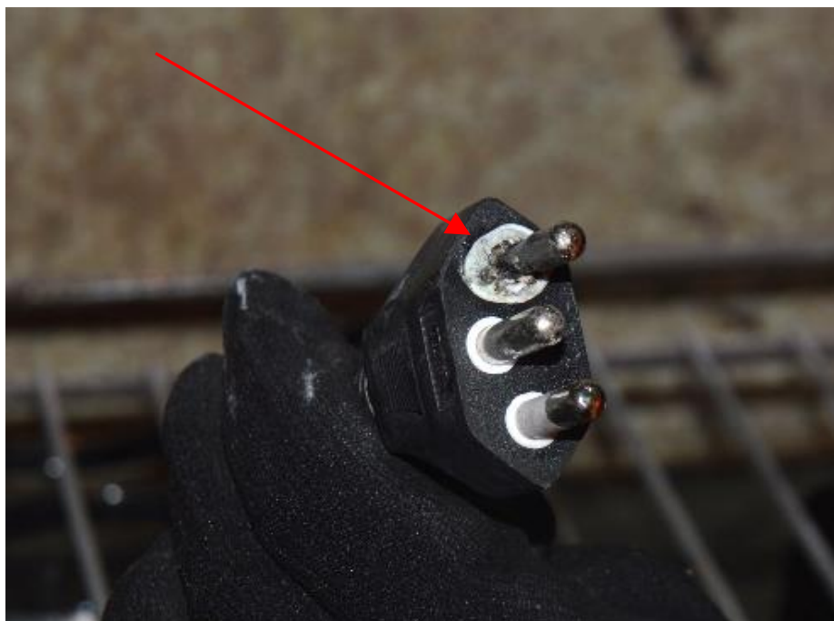
Figura 85 - A seta indica a ocorrência de um fenômeno termelétrico em um dos plugs da tomada
