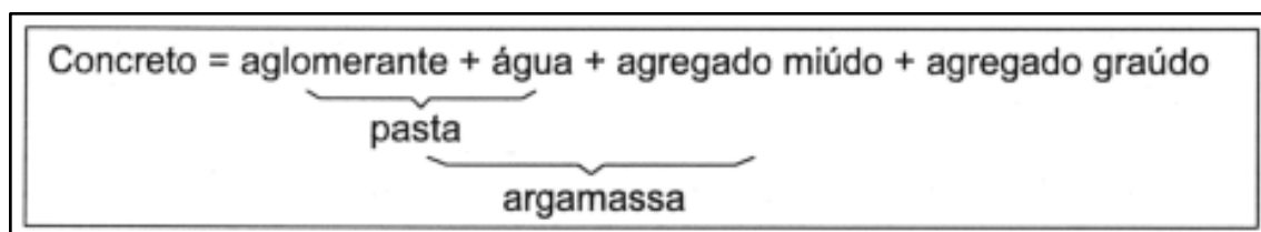
Figura 60 - Traço de concreto
