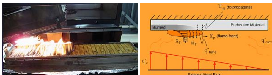
Figura 22 - Aparato de teste da ASTM E 1321
