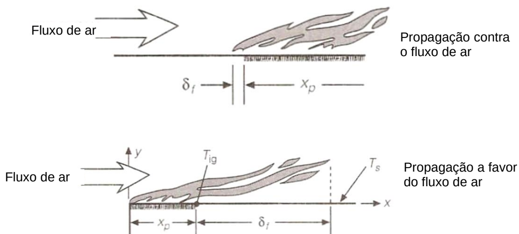
Figura 21 - Propagação lateral da chama a favor e contra o fluxo de ar
