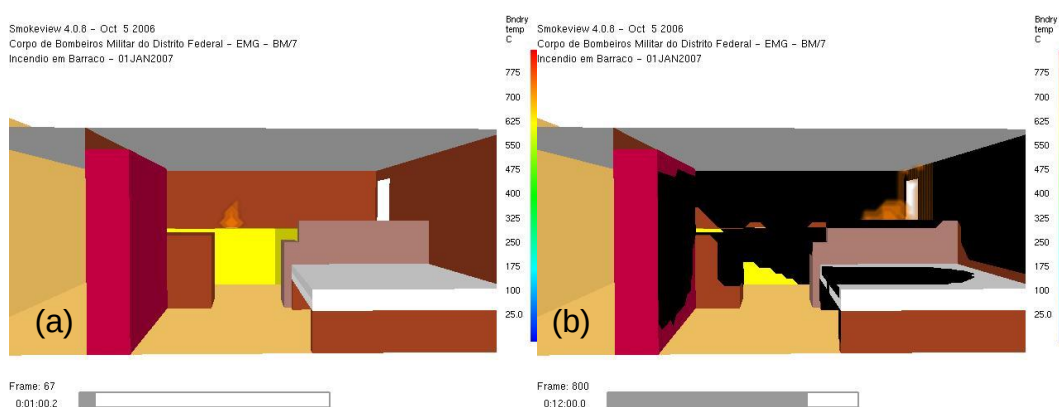
Figura 46 - Influência da ventilação nas marcas de queima. Simulação computacional realizada em um incêndio real periciado pelo CBMDF
