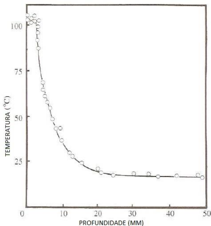
Figura 7 - Gráfico da temperatura do líquido em função da profundidade
