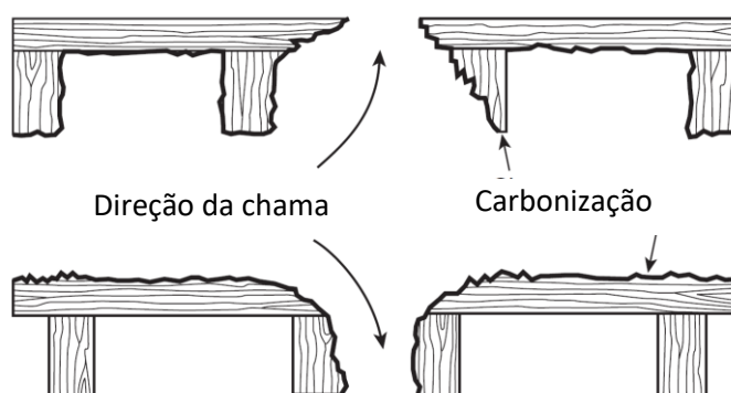
Figura 41 - Degradação da superfície horizontal do mobiliário
