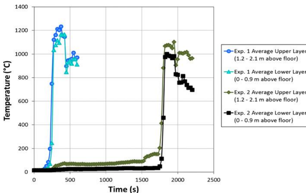
Figura 29 - Gráfico da média entre a temperatura nas camadas superiores e inferiores nos ambientes com mobiliário novo (experimento 1) e antigo (experimento 2)
