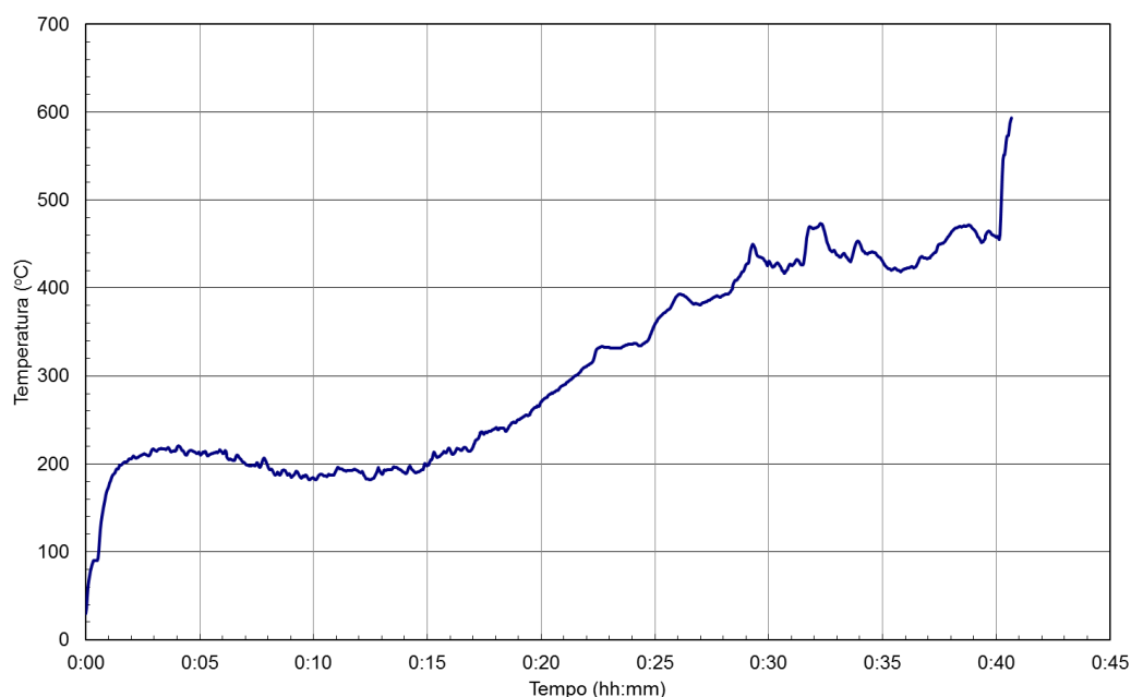
Figura 18 - Gráfico da evolução da temperatura em uma placa de papel prensado devido à queima de um cigarro
