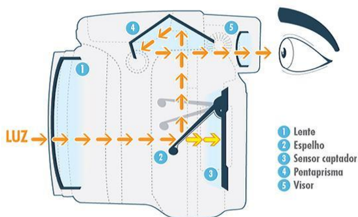
Figura 143 - Espelhos que reduzem o erro de paralaxe nas câmeras digitais
