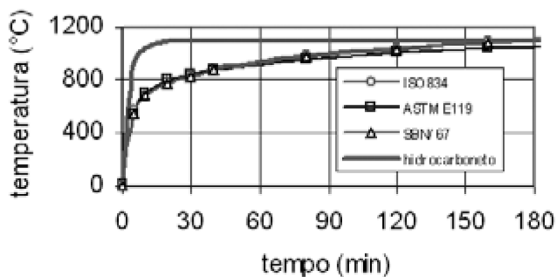
Figura 67 - Curva padrão de hidrocarbonetos
