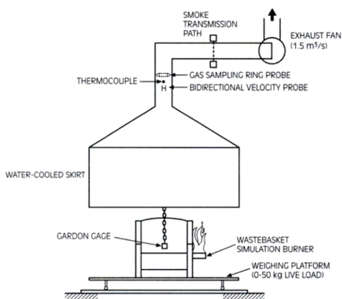
Figura 24 - Representação esquemática de um cone calorímetro
