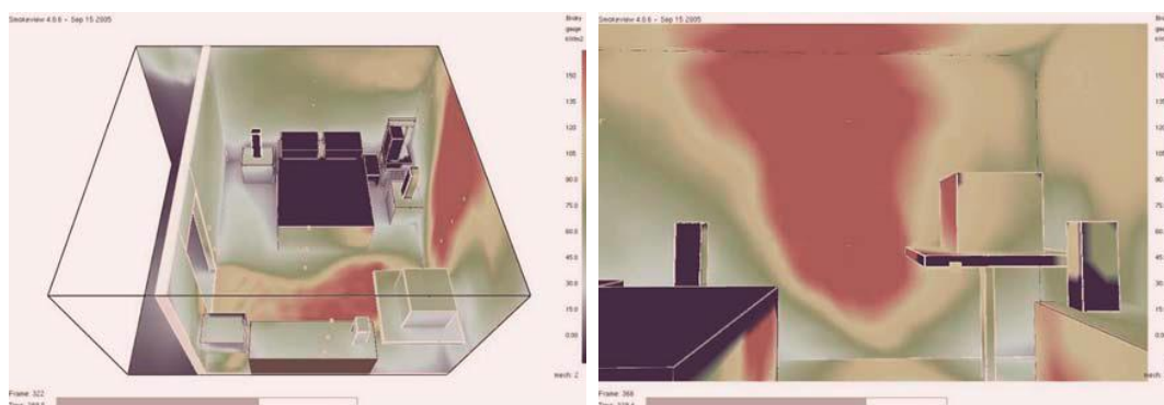
Figura 51 - Perfil do fluxo de calor nas superfícies 12 segundos após a generalização do incêndio ( flashover ) debelado após 2 minutos e 30 segundos
