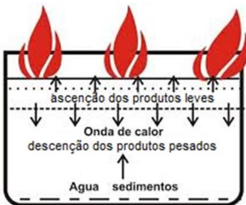
Figura 8 - esquema da zona quente se propagando pelo tanque até atingir a água depositada no fundo e causar o boilover
