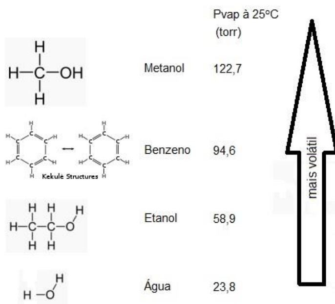
Figura 11 - exemplificação da relação entre pressão de vapor e volatilidade
