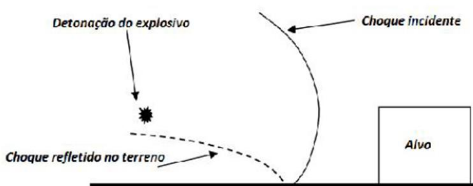
Figura 112 - Esquema da propagação de uma onda de choque devido a uma explosão acima do nível do solo
