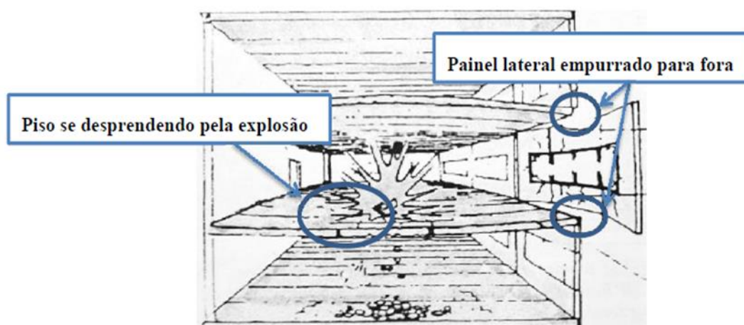
Figura 124 - Esquema de uma explosão interna resultando em colapso progressivo, tendo o comportamento da propagação da onda de choque em estruturas com diferentes geometrias
