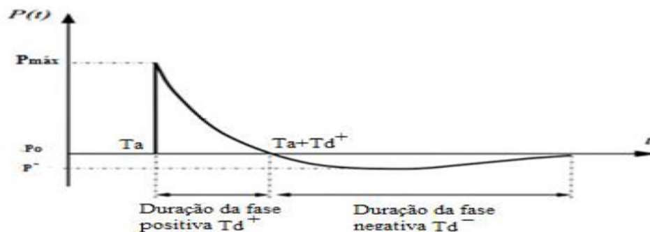
Figura 111 - Gráfico da pressão típica em função do tempo de uma onda de choque
