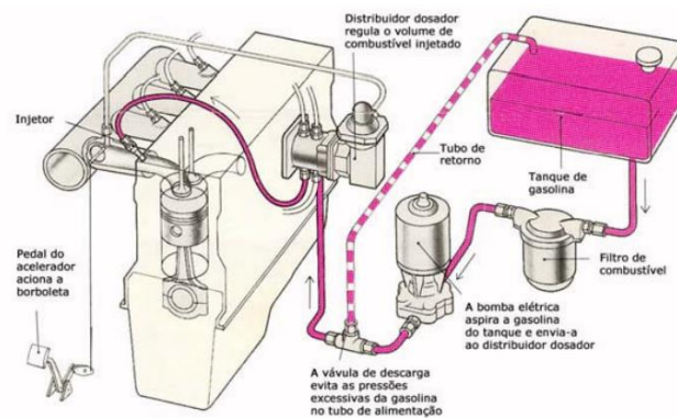
Figura 41 - Esquema do sistema de alimentação do combustível até o bico injetor
