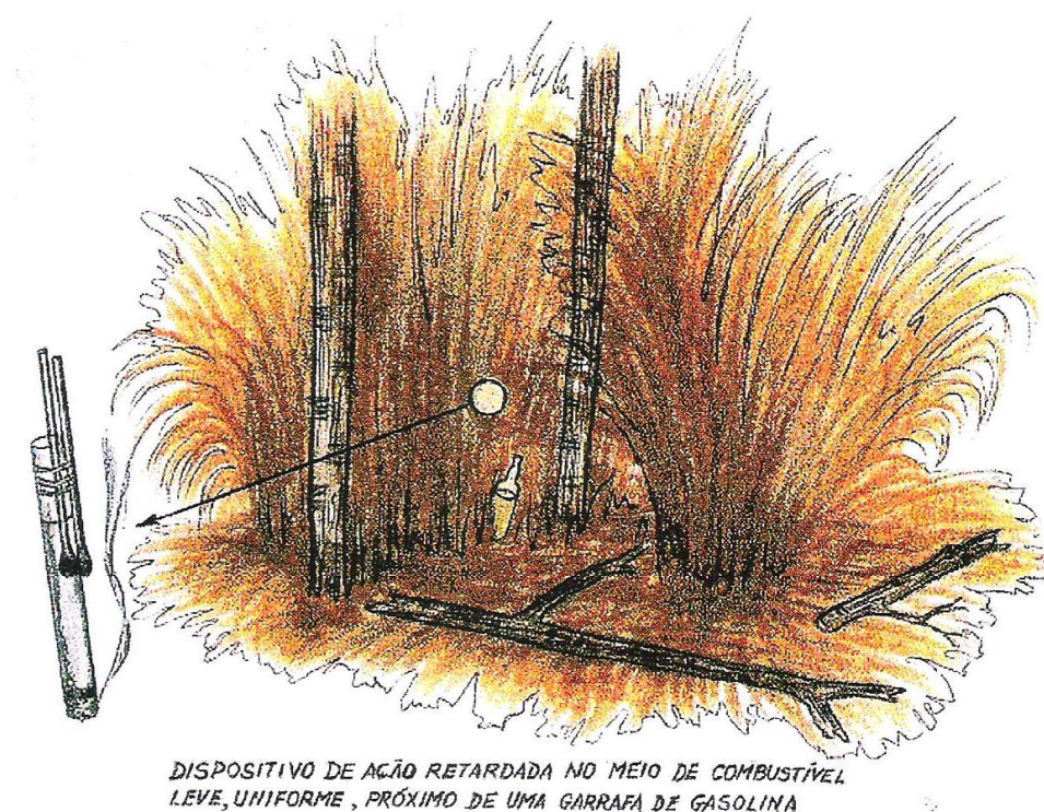
Figura 91 - Exemplo de dispositivo de ação retardada
