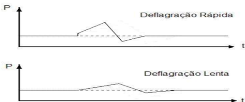
Figura 107 - Exemplos de comportamentos de deflagrações do ponto de vista de um alvo
