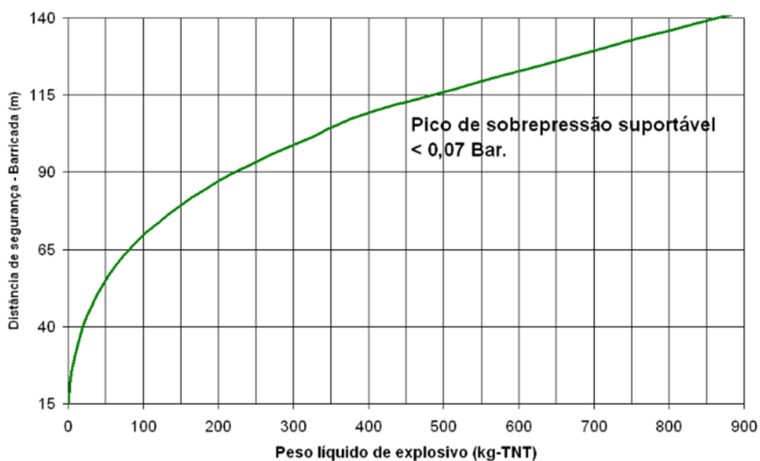
Figura 126 - Distância de segurança contra os efeitos diretos da onda de choque sobre o homem
