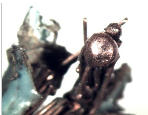
Figura 15 - Traço de fusão por curto-circuito
