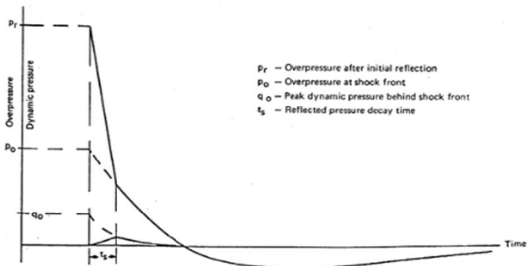
Figura 119 - Sobrepressão e pressão dinâmica em função do tempo, passando por uma estrutura esférica
