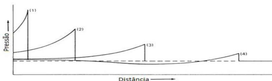
Figura 109 – Curva típica da pressão x distância de uma explosão
