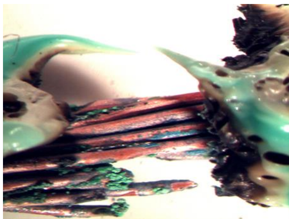
Figura 25 - Fenômeno elétrico de desconexão parcial
