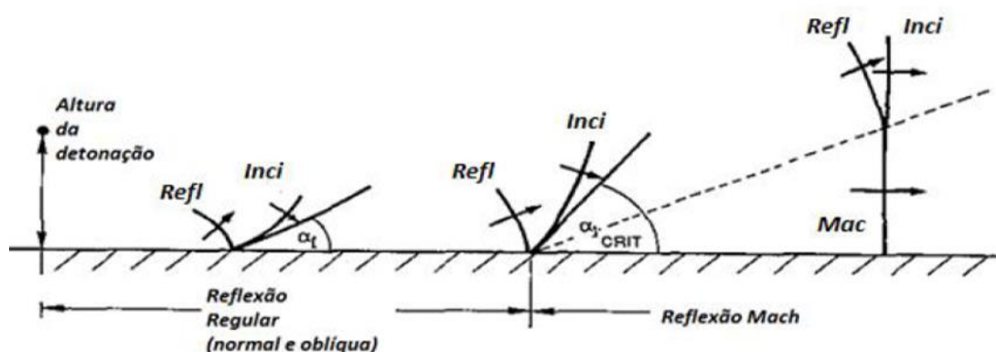
Figura 115 - Interação de uma onda de choque com uma superfície, para diferentes sentidos de propagação
