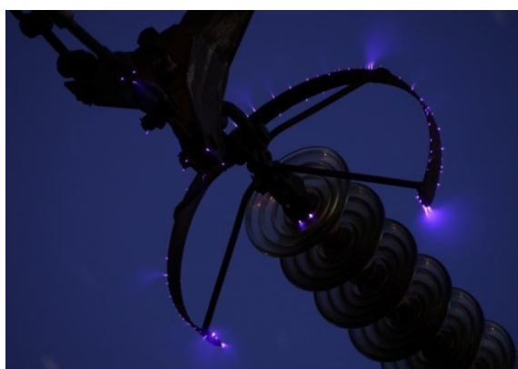
Figura 38 - Efeito corona em uma rede de alta tensão
