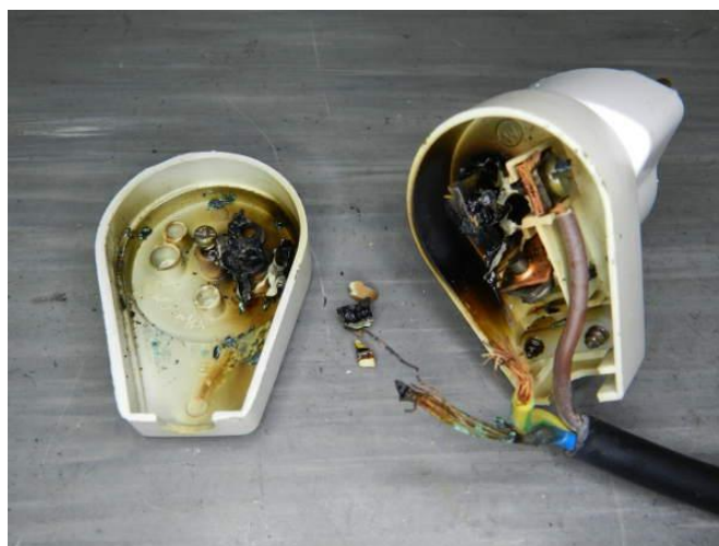
Figura 33 - Contato imperfeito em tomada
