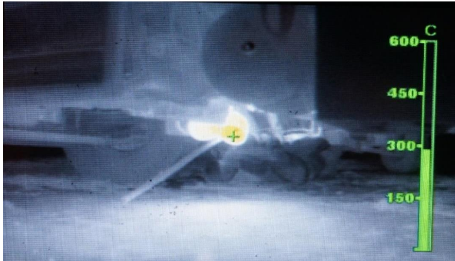
Figura 40 - O escapamento da viatura do CBMDF, motor diesel, chegou a 320°C, medido com termopares
