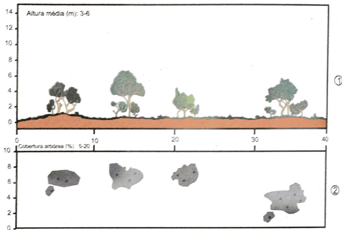
Figura 59 - Parque de cerrado, também chamado de campo de murunduns
