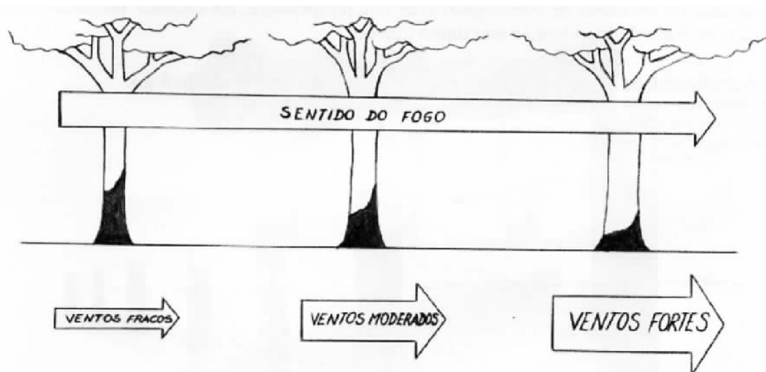
Figura 85 – Influência da intensidade do vento na altura de carbonização
