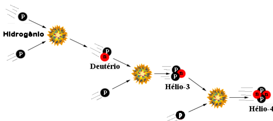
Figura 102 - Fusão Nuclear
