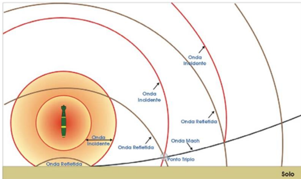
Figura 114 - Efeito da detonação no ar formando onda mach
