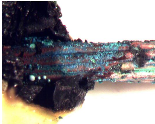
Figura 30 - Perda de propriedade física do fio condutor
