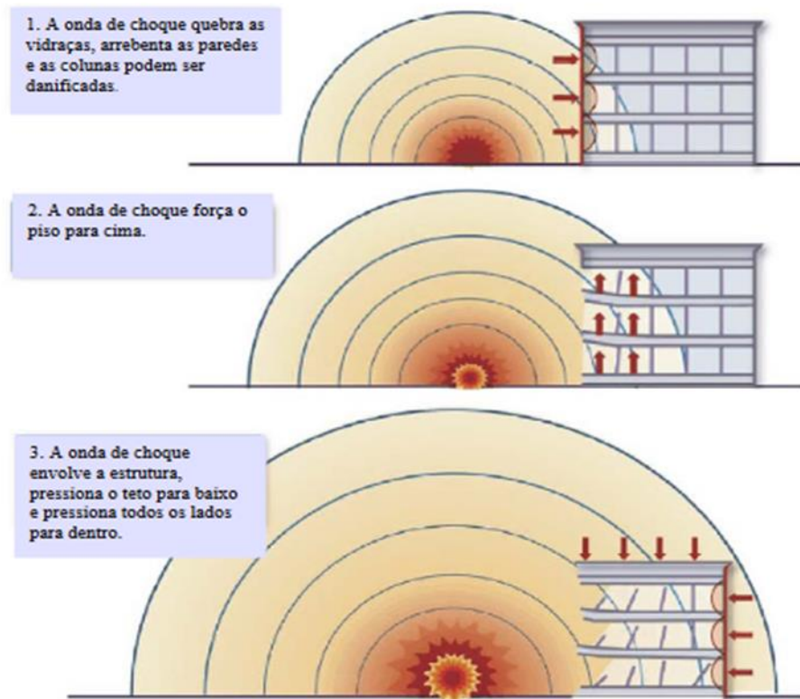
Figura 121 - Estrutura submetida a carregamento por difração
