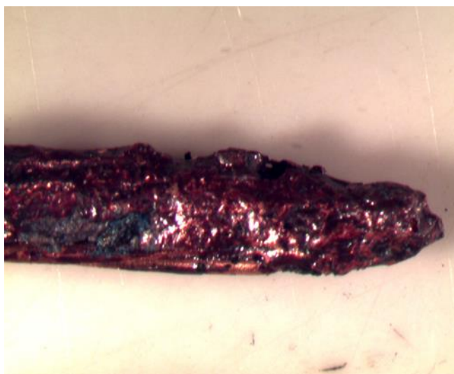
Figura 21 - Traço de fusão de sobrecarga com ruptura
