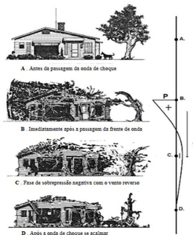
Figura 110 - Caso genérico ilustrativo das fases de uma explosão e seus efeitos sobre estruturas alvos.
