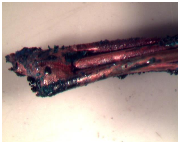
Figura 29 - Traço de fusão de sobrecarga com ruptura
