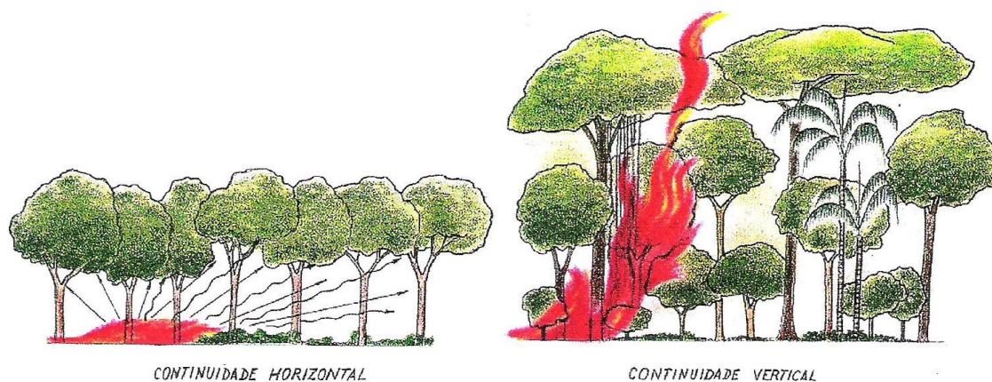
Figura 70 - Continuidade de vegetação
