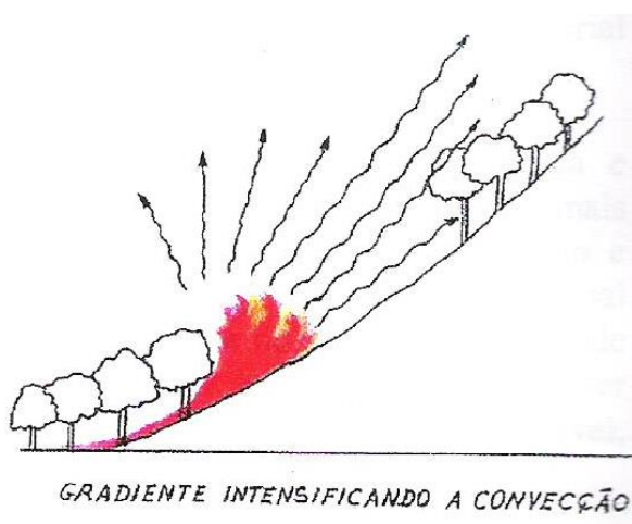
Figura 74 - Terreno em aclive, cuja propagação do incêndio segue a inclinação, intensificando o fenômeno da convecção
