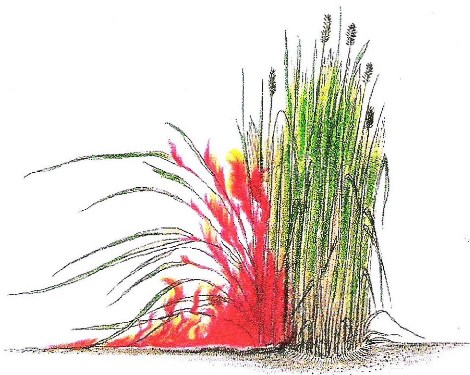
Figura 78 - Gramíneas sujeitas ao fogo sem vento
