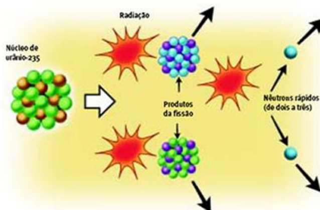
Figura 101 - Fissão Nuclear
