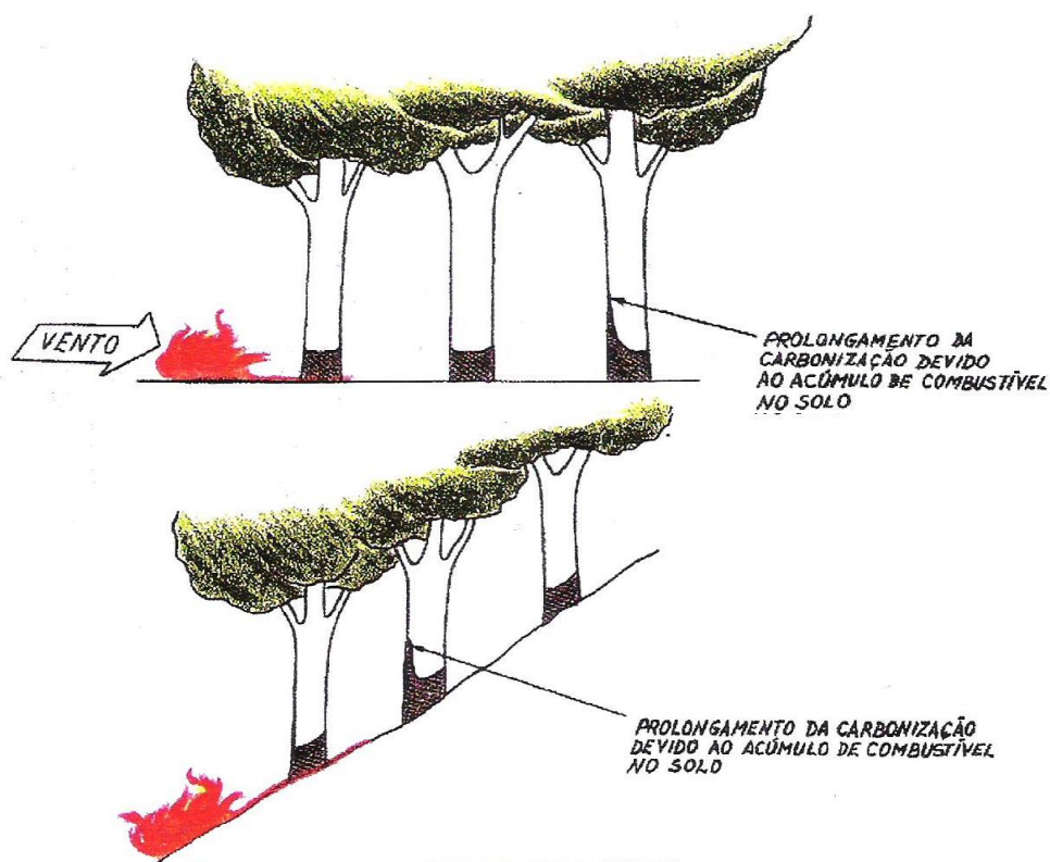
Figura 84 - Queima morro abaixo ou num plano horizontal contra o vento
