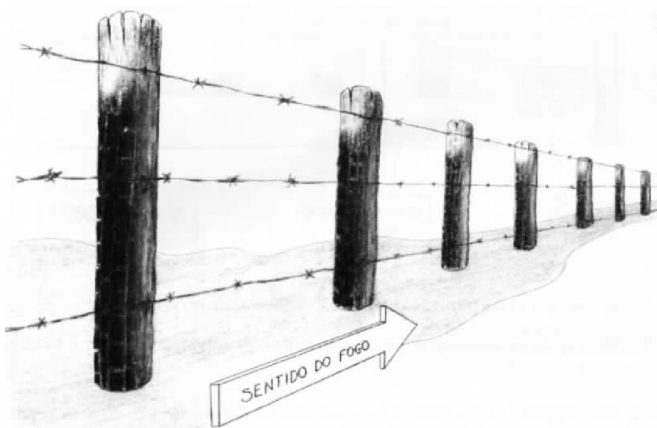
Figura 87 - Carbonização em forma de escamas de jacaré
