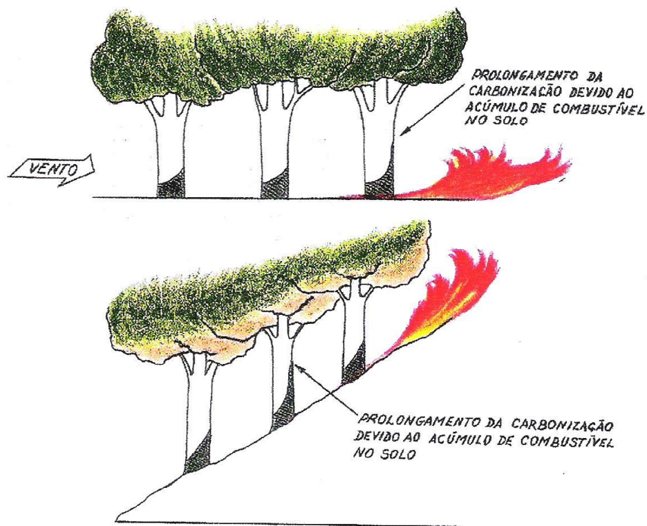
Figura 82 - Queima morro acima ou num plano horizontal a favor do vento
