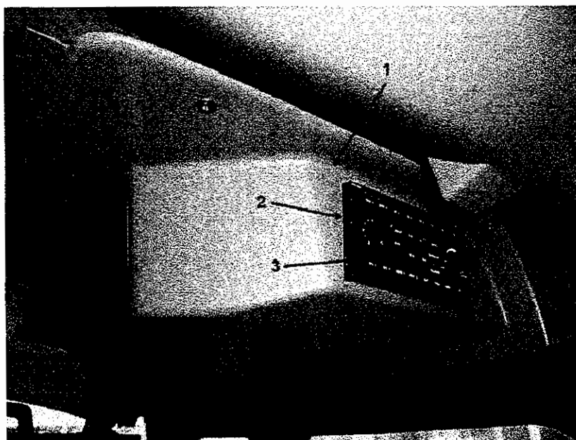
Figure 3: 3ª e/ou 4ª Unidade Comando de Áudio ACU 6100 para membro da tripulação da cabine – instalação traseira
