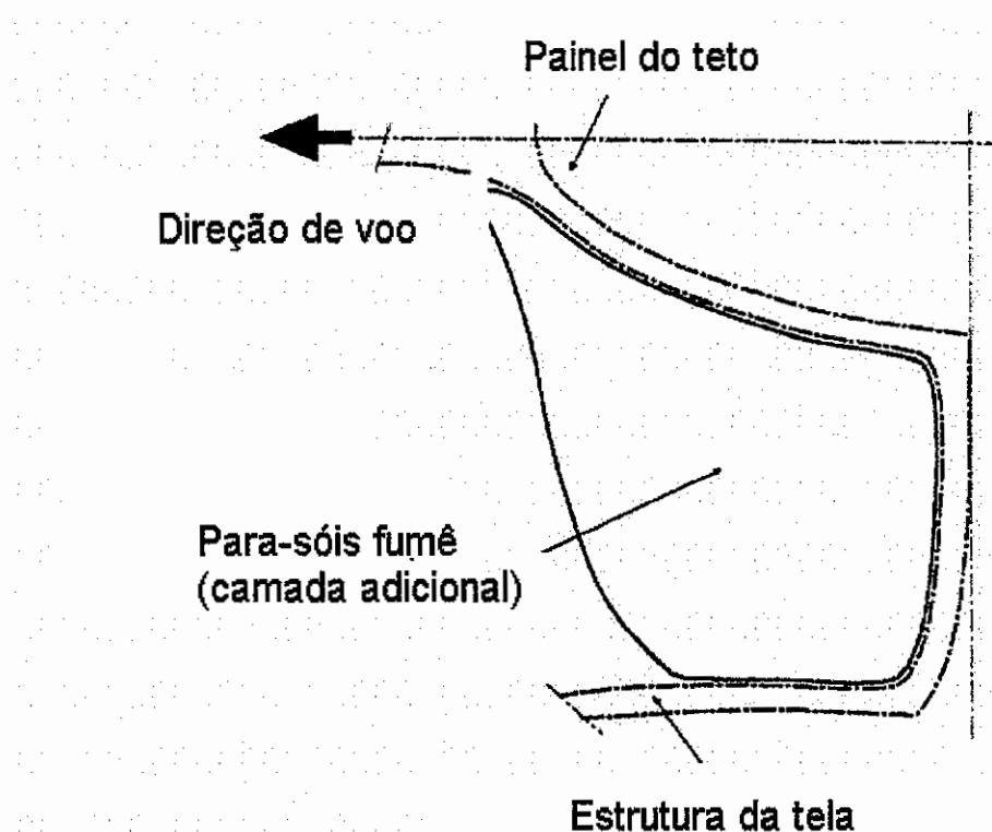
Figura 1: Para-sóis fumê para a parte superior do para-brisa do posto de pilotagem - exemplo
