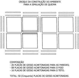
Figura 2. Croqui modelo de construção de simulador com paredes
