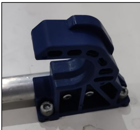
Figura 9 – Sistema de retenção dianteiro esquerdo após os ensaios
